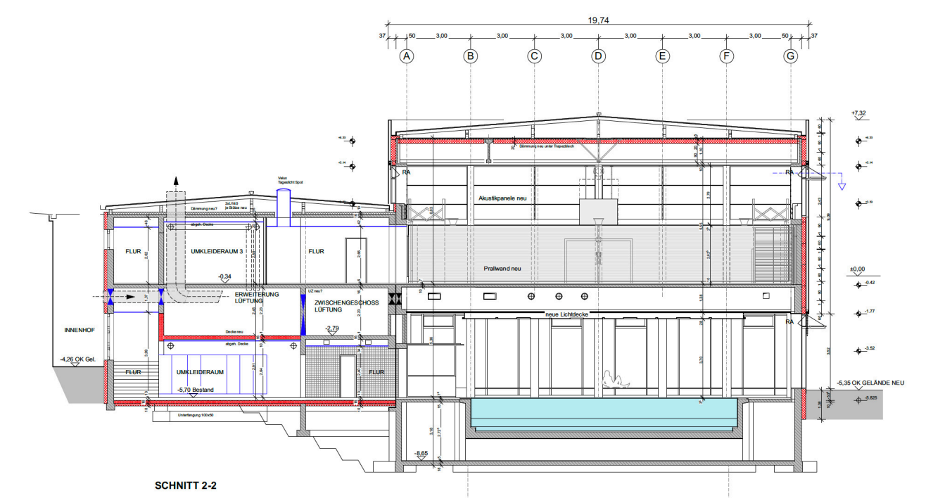
Querschnitt Schwimm- und Turnhalle © Arch.
